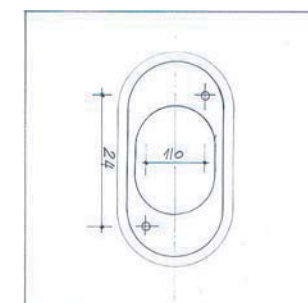
Scellement vue en plan
