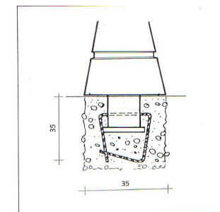
Scellement
